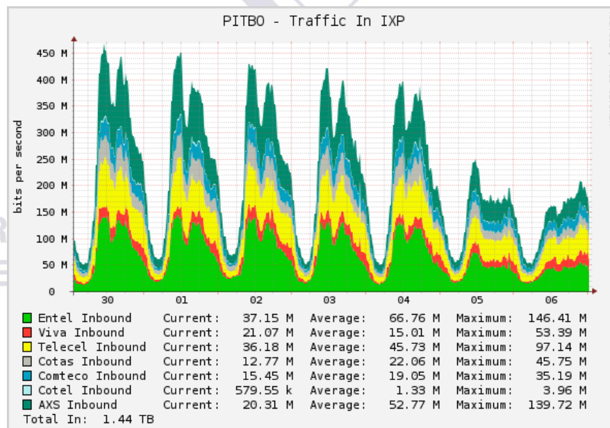
Figura 6 - Tráfico última semana entrada al PIT
